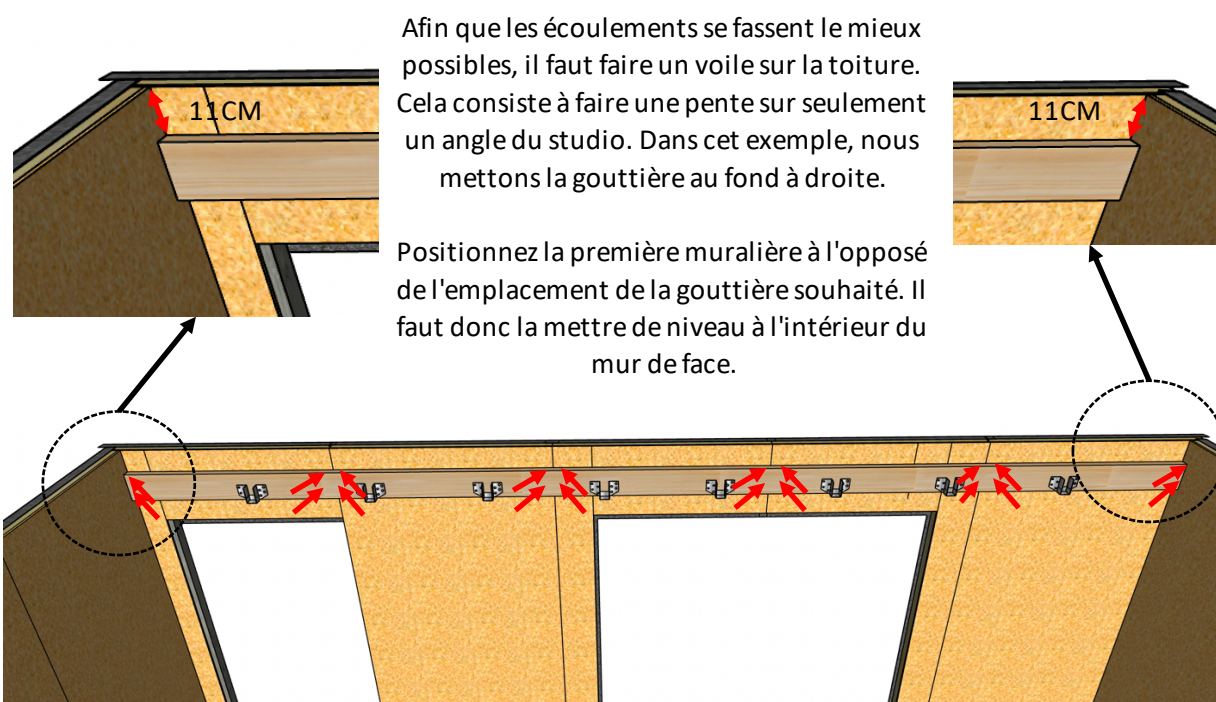
Fixation de la première muralière sans pente
